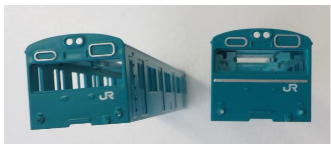
▼低運転台車と高運転台車
